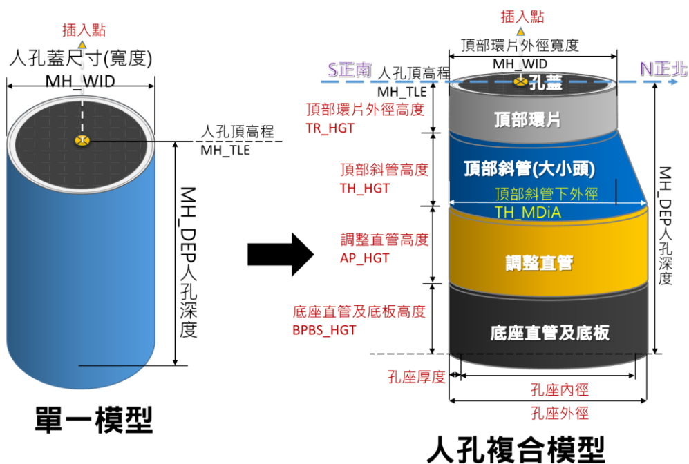
圖 1.2 污水下水道人孔 3D 模型示意圖
